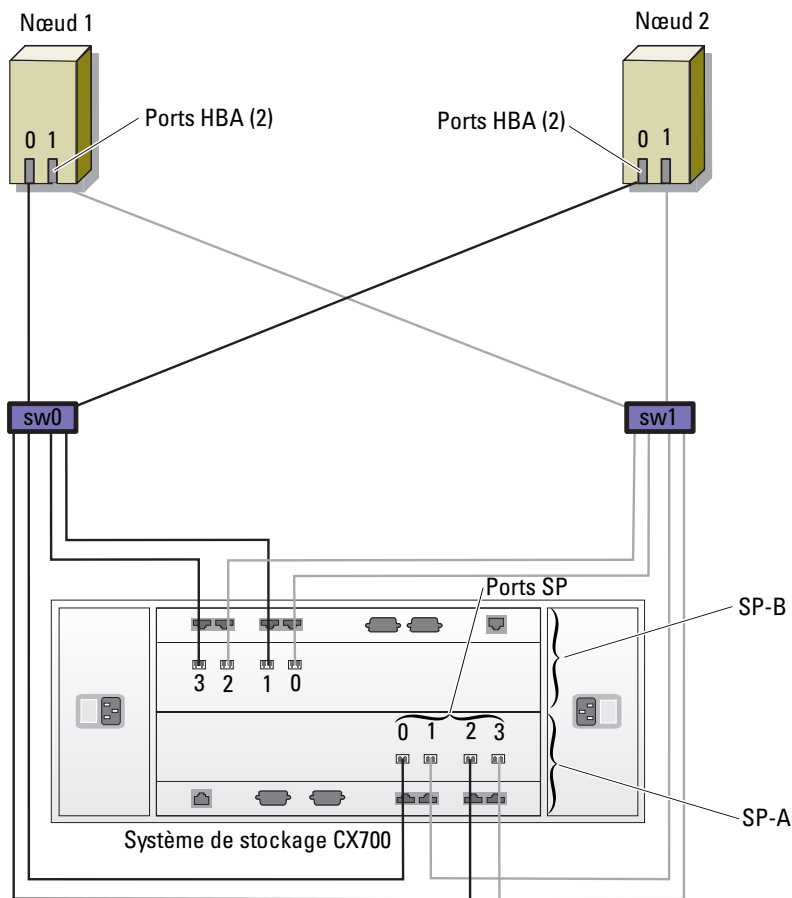
Figure 1-3. Câblage dans un cluster Fibre Channel connecté à un SAN
